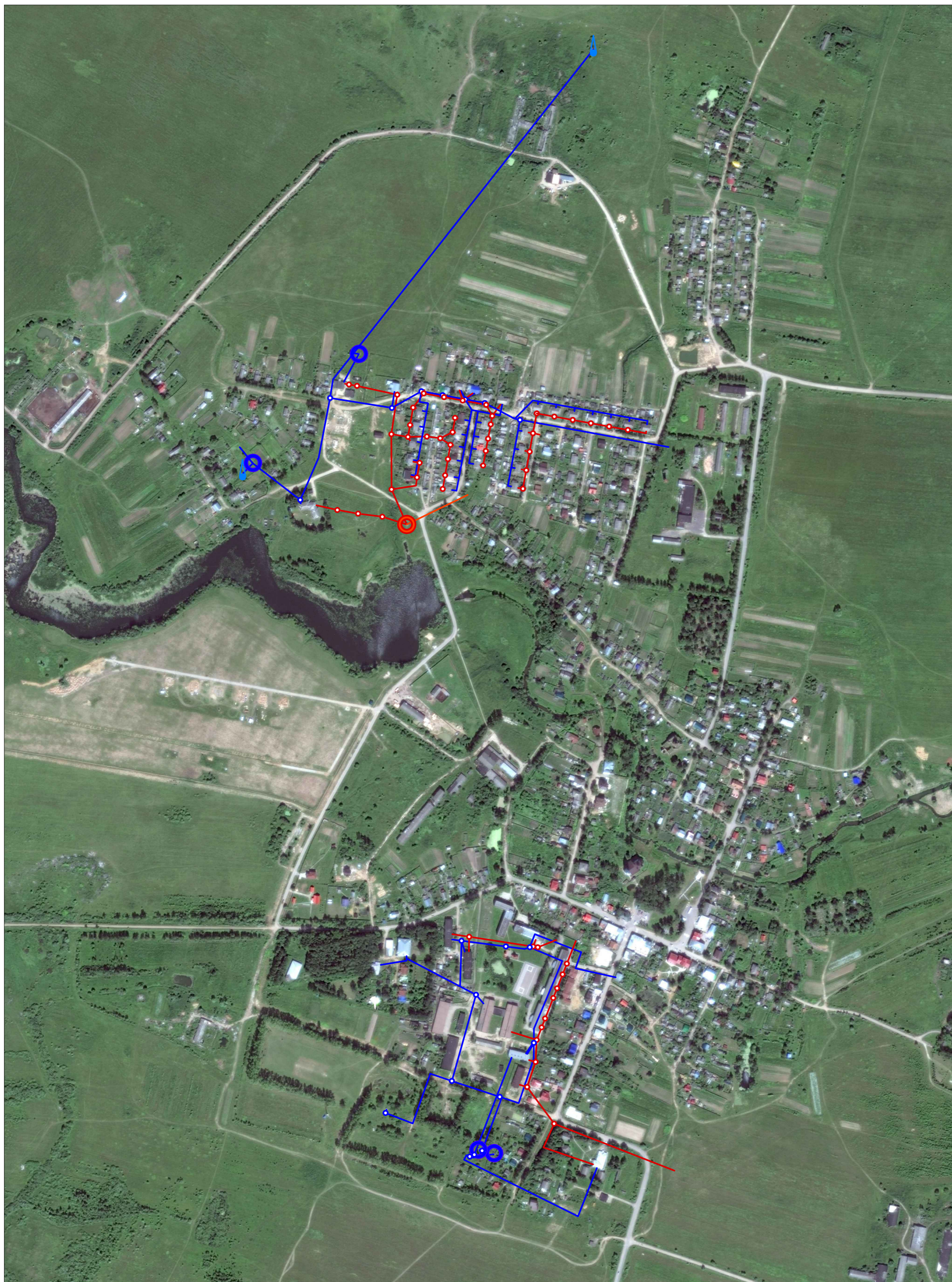
Схема водоснабжения и водоотведения с. Вятское и д. Кондреево - фрагмент территории М 1:5 000
